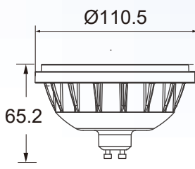
Base Type : GU10
