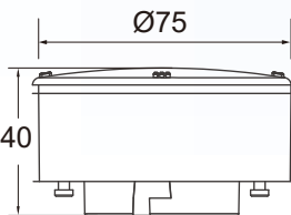
Base Type : GX53
