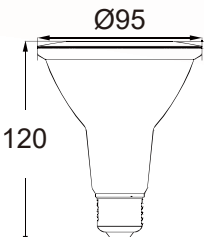
Base Type : E26
